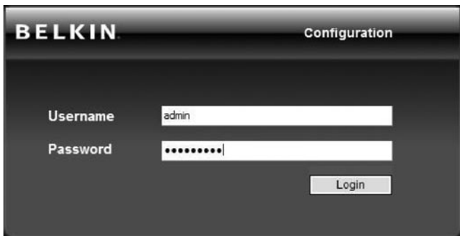
Fig. 1 Login Page
